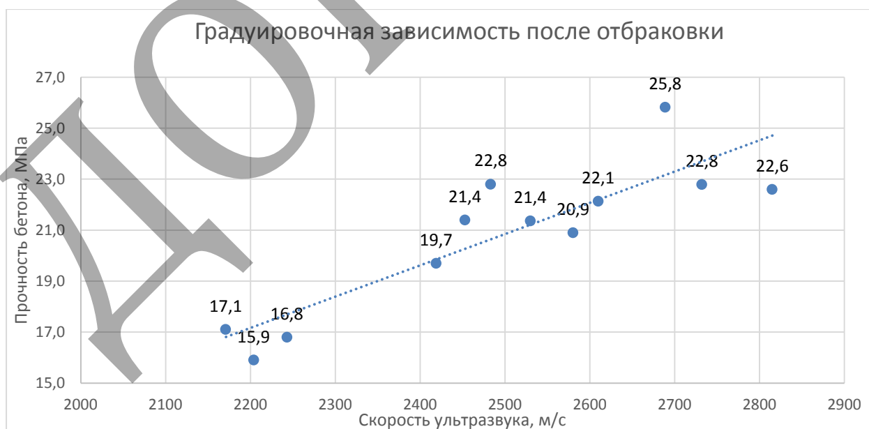
Рисунок 3.5 – График градуировочной зависимости после отбраковки
