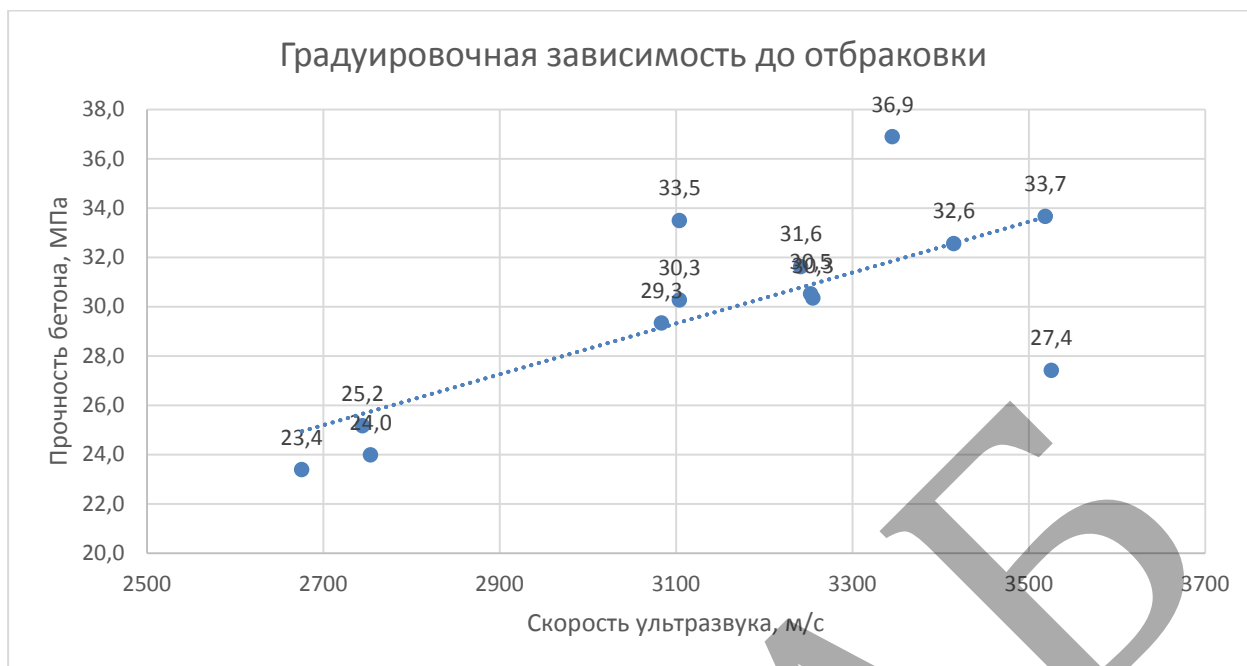
Рисунок 3.7 – График градуировочной зависимости до отбраковки
