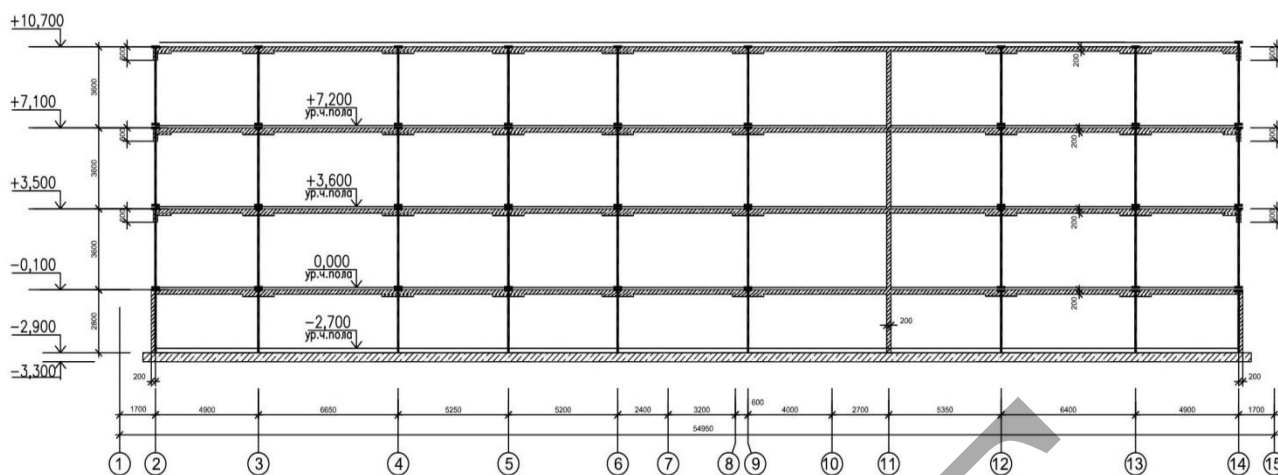
Рисунок 3.2 – Разрез 1-1
