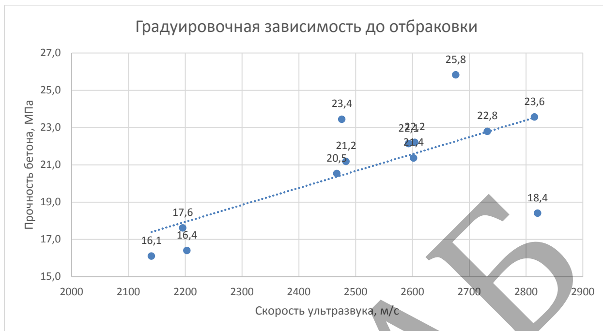
Рисунок 3.10 – График градуировочной зависимости до отбраковки
