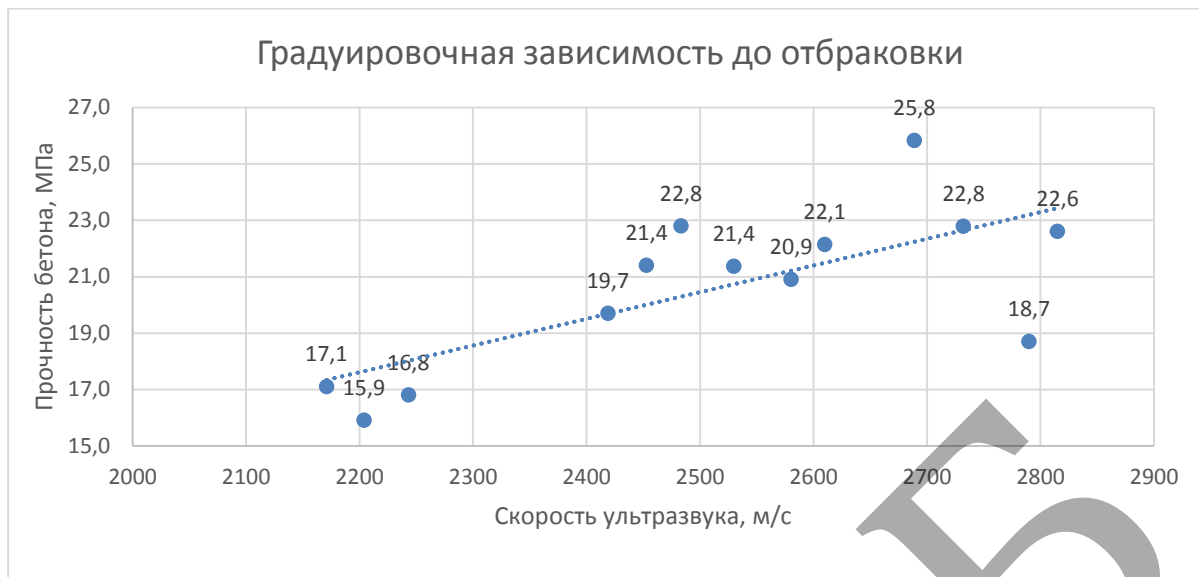
Рисунок 3.4 – График градуировочной зависимости до отбраковки
