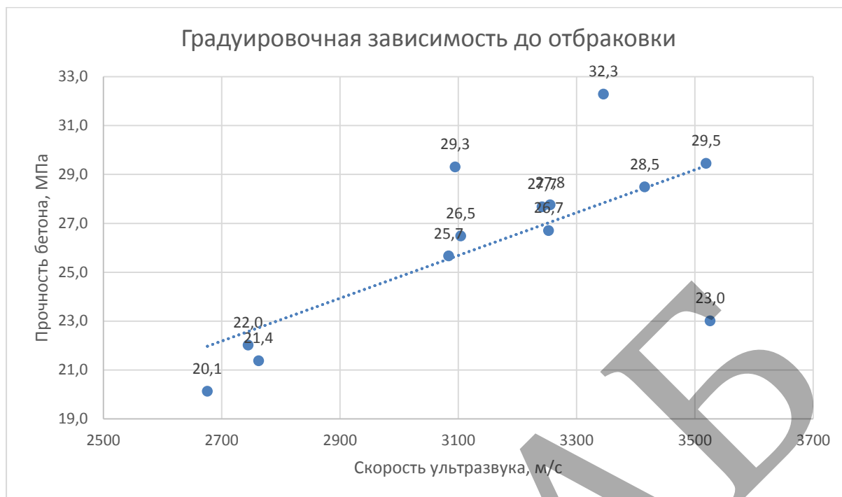
Рисунок 3.13 – График градуировочной зависимости до отбраковки
